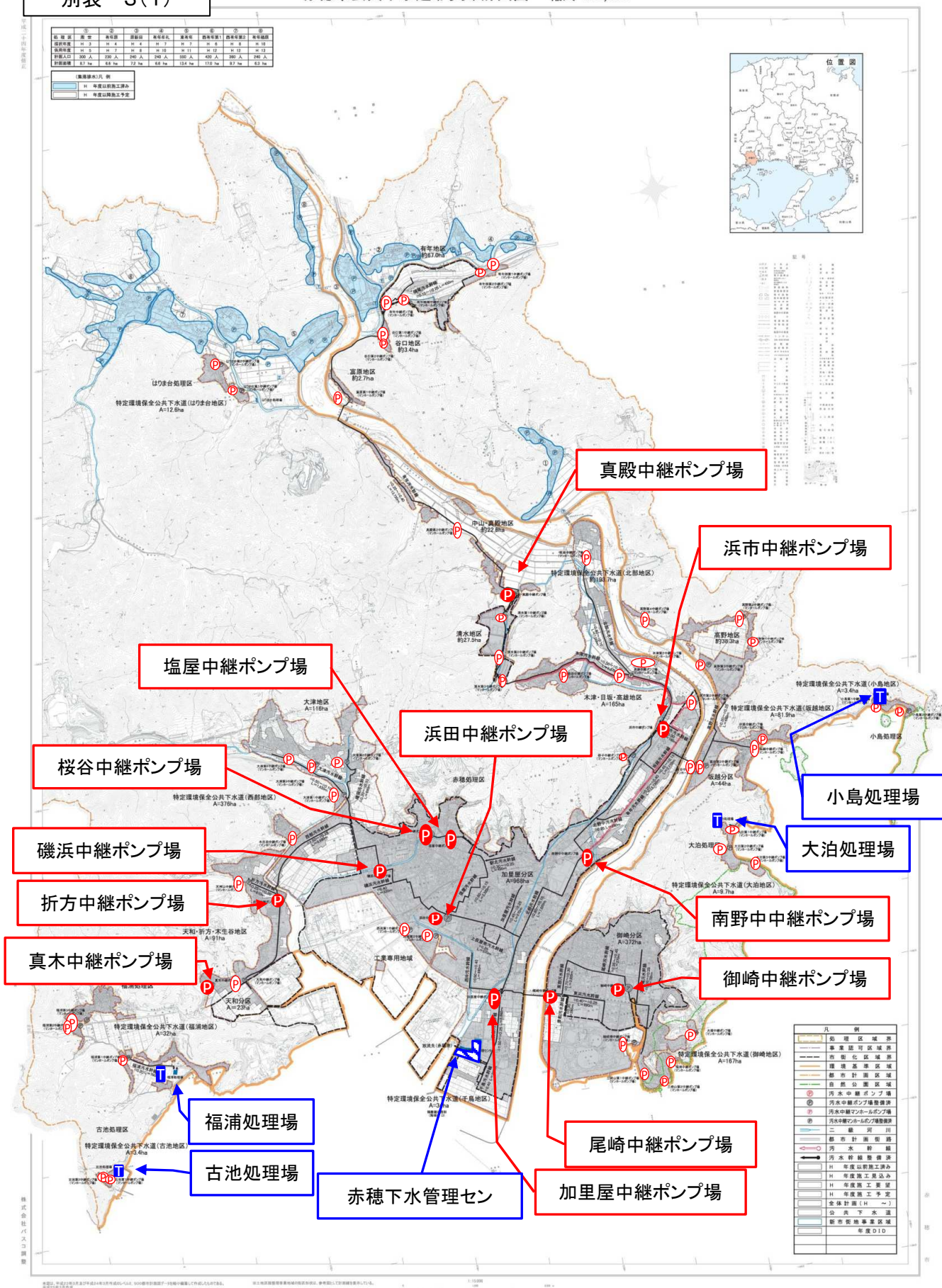
赤穂市公共下水道(汚水)計画図 縮尺 1:15,000
