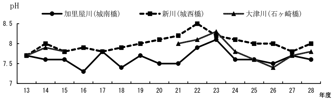
図5-1-2 市内小河川の水質経年変化（最下流地点）
